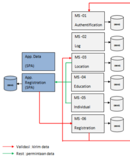
Gambar 2. Rancangan sistem informasi menggunakan microservice
