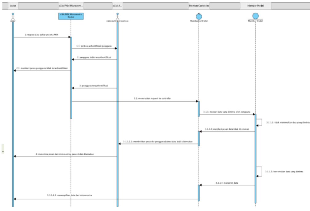
Gambar 4 . Alur sistem xSIA PKM menggunakan microservice
