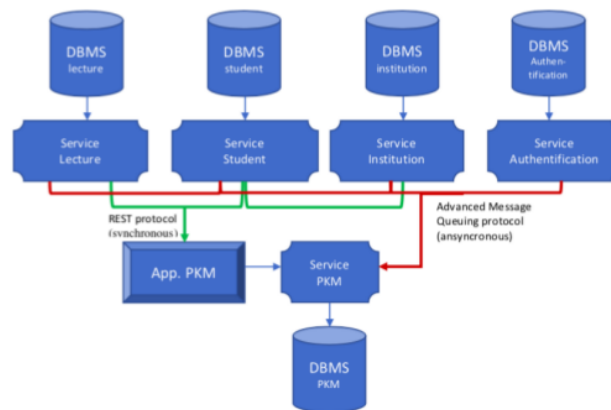
Gambar 3. Arsitektur Microservice xSIA PKM
