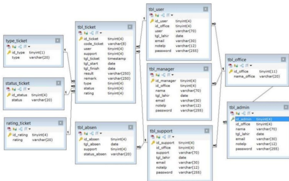
Gambar 3. ERD
