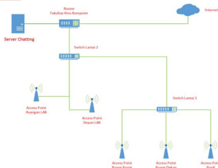
Gambar 2. Perancangan topologi jaringan intranet server chatting
