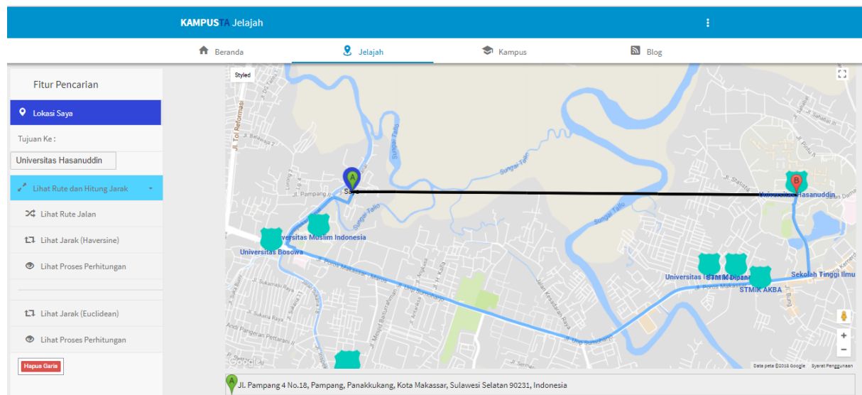
Gambar 2. Halaman Jelajah
