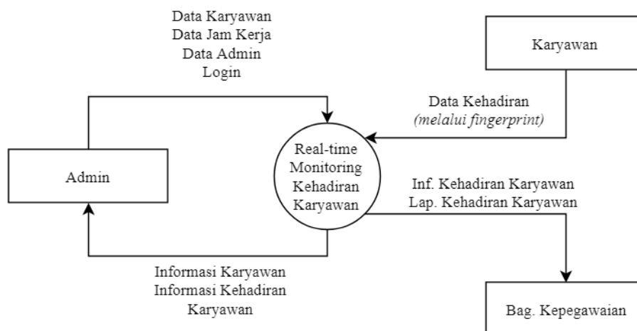
Gambar 2. Diagram Konteks
