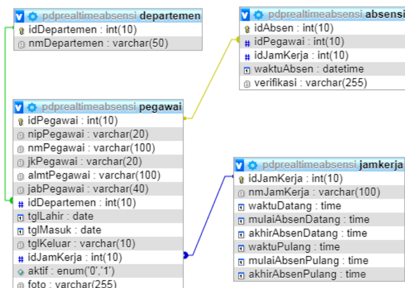
Gambar 3. Relasi Tabel
