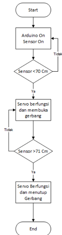
Gambar 3 Flowchart sistem kontrol pintu gerbang otomatis
