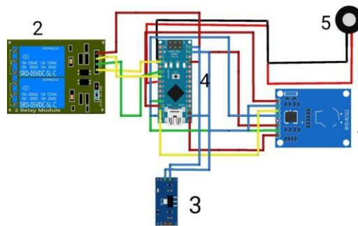
Gambar 9. Rangkaian elektronik
